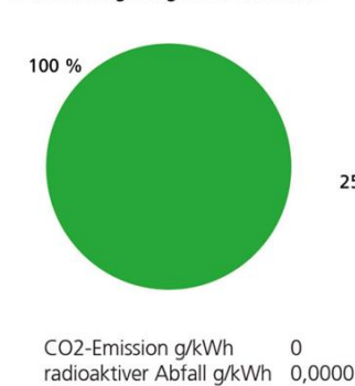
Gesamtenergieträgermix GWN 2023
