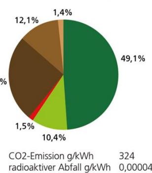
Strommix Deutschland 2023 2)
