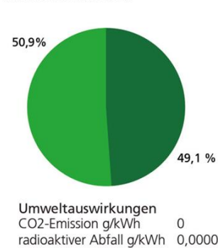
Produktmix GWN 2023
